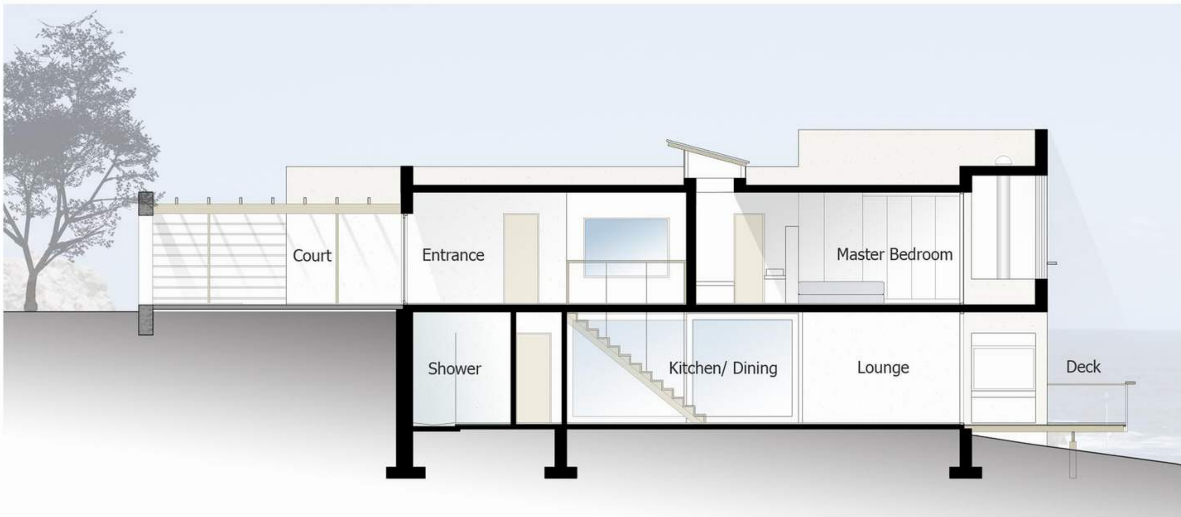
TYPICAL SECTION n.t.s.
