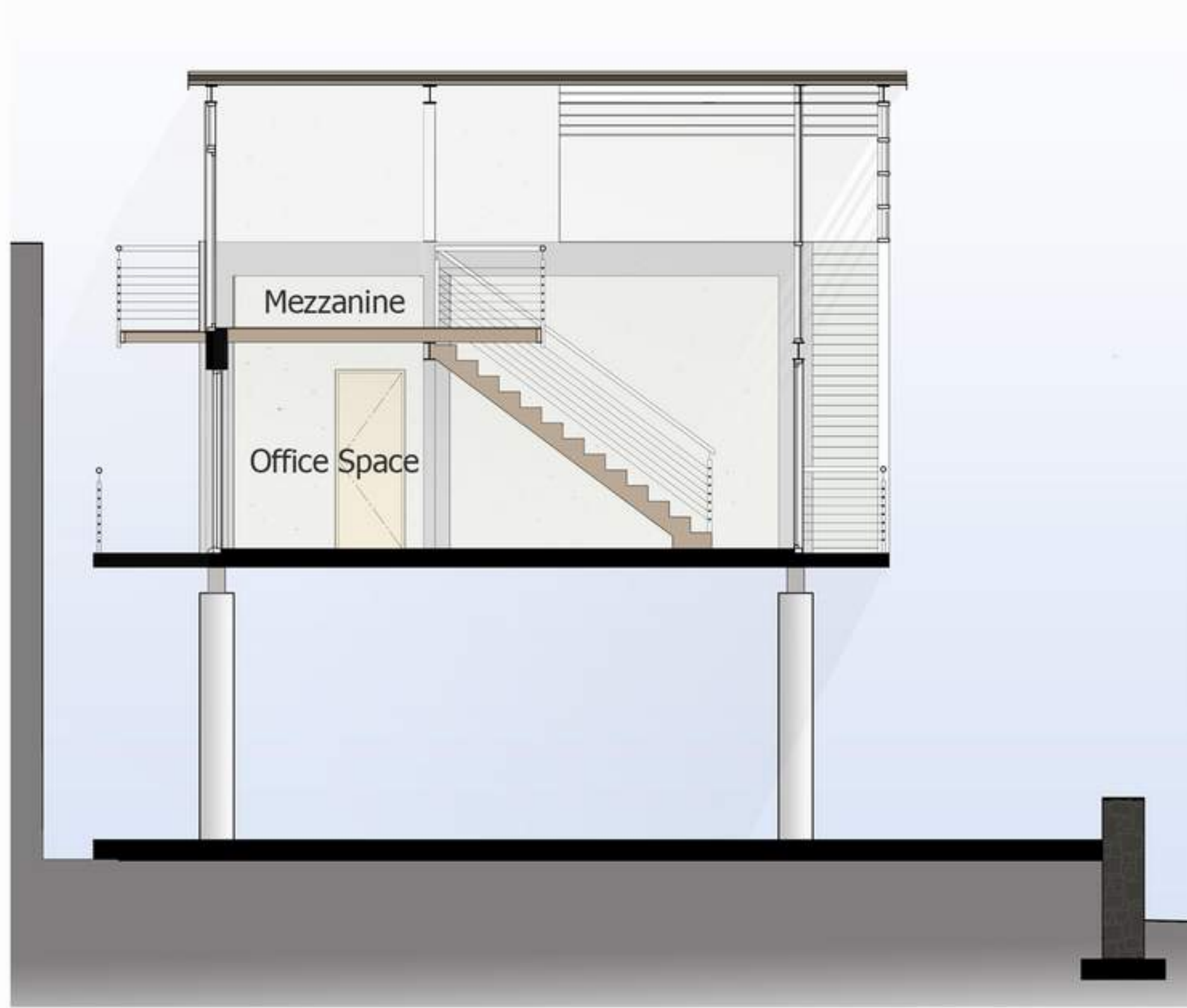
TYPICAL SECTION n.t.s.
