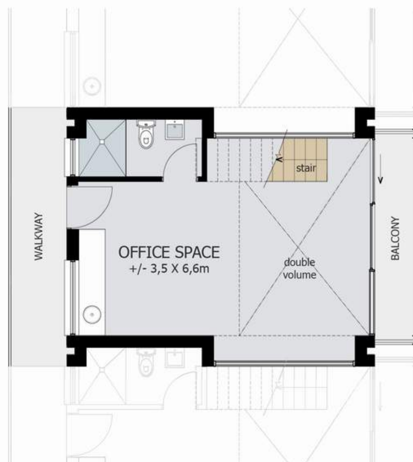
LEVEL 1 n.t.s.
