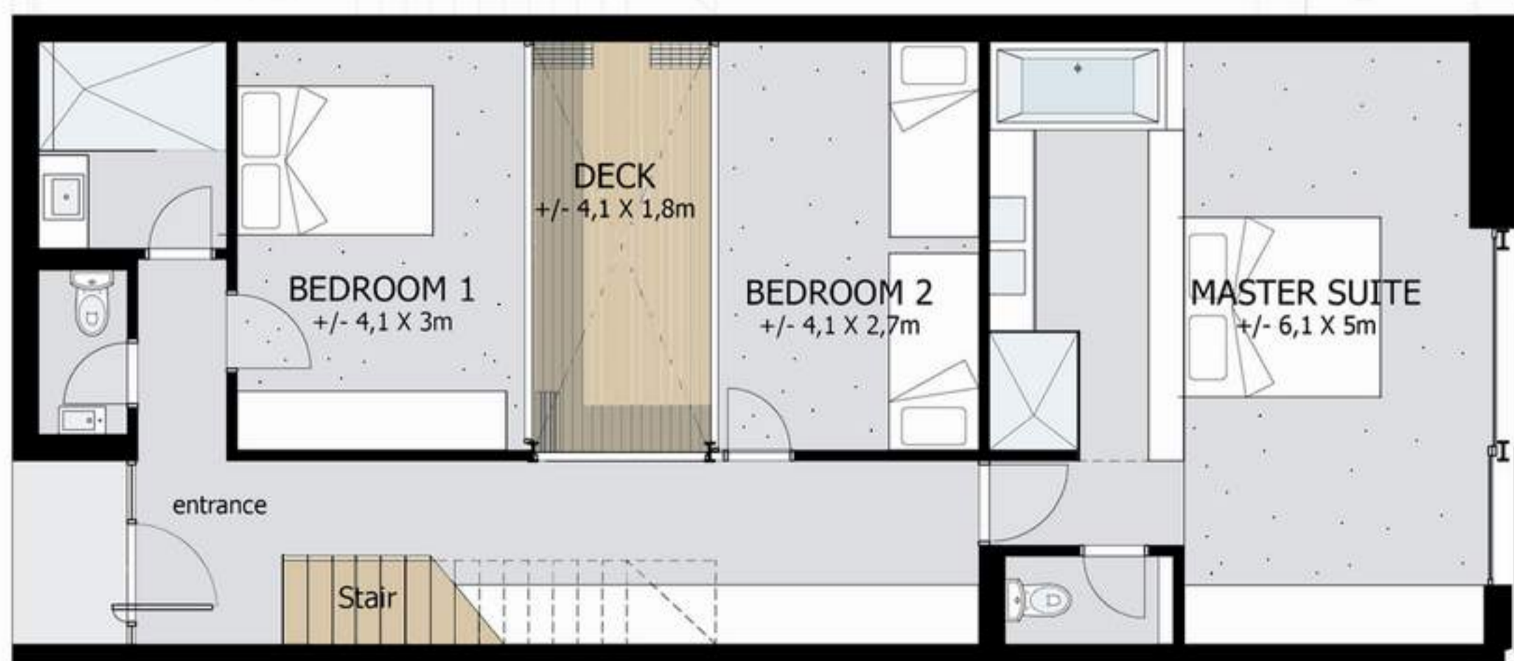
LEVEL 1 n.t.s.
