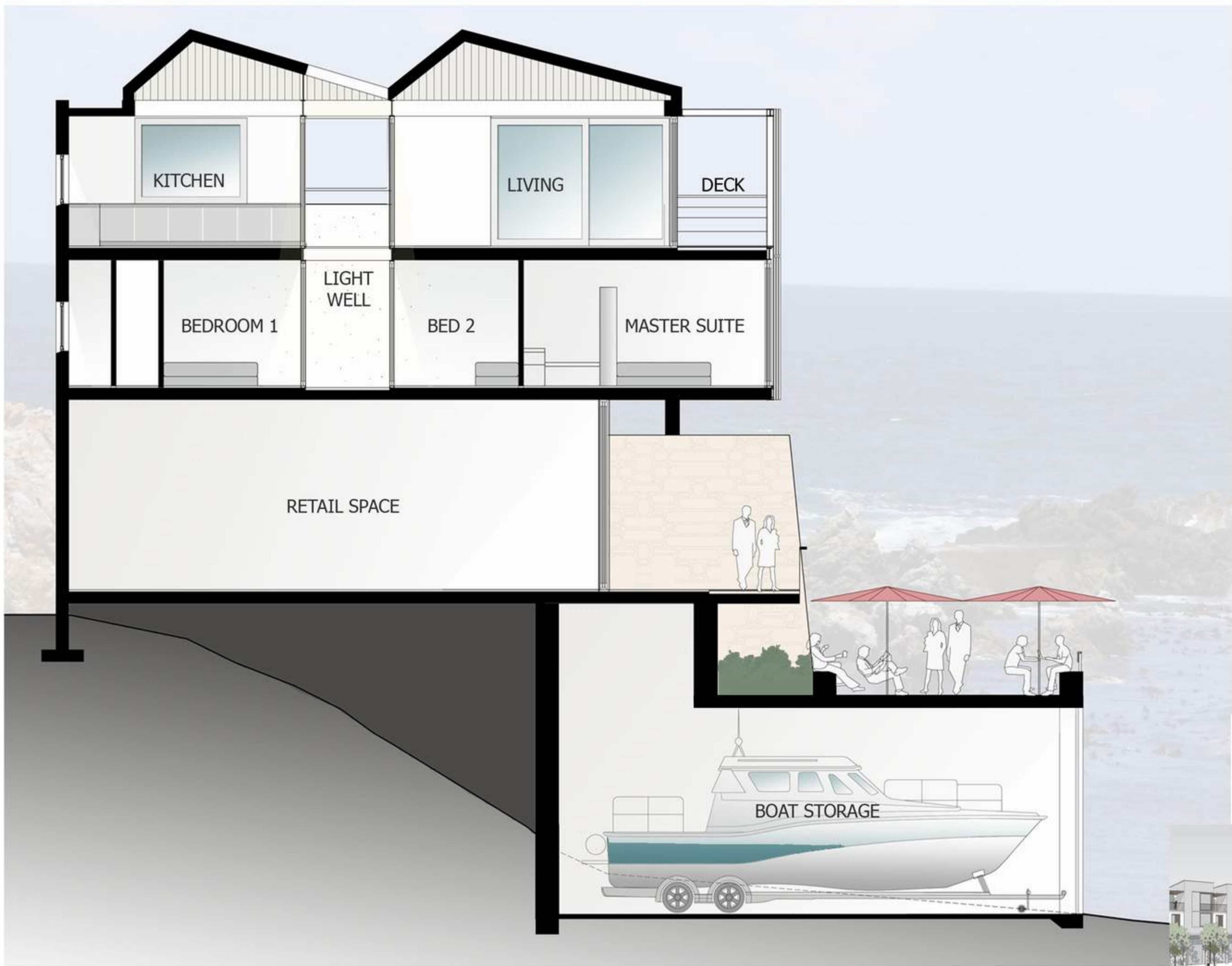
TYPICAL SECTION n.t.s.
