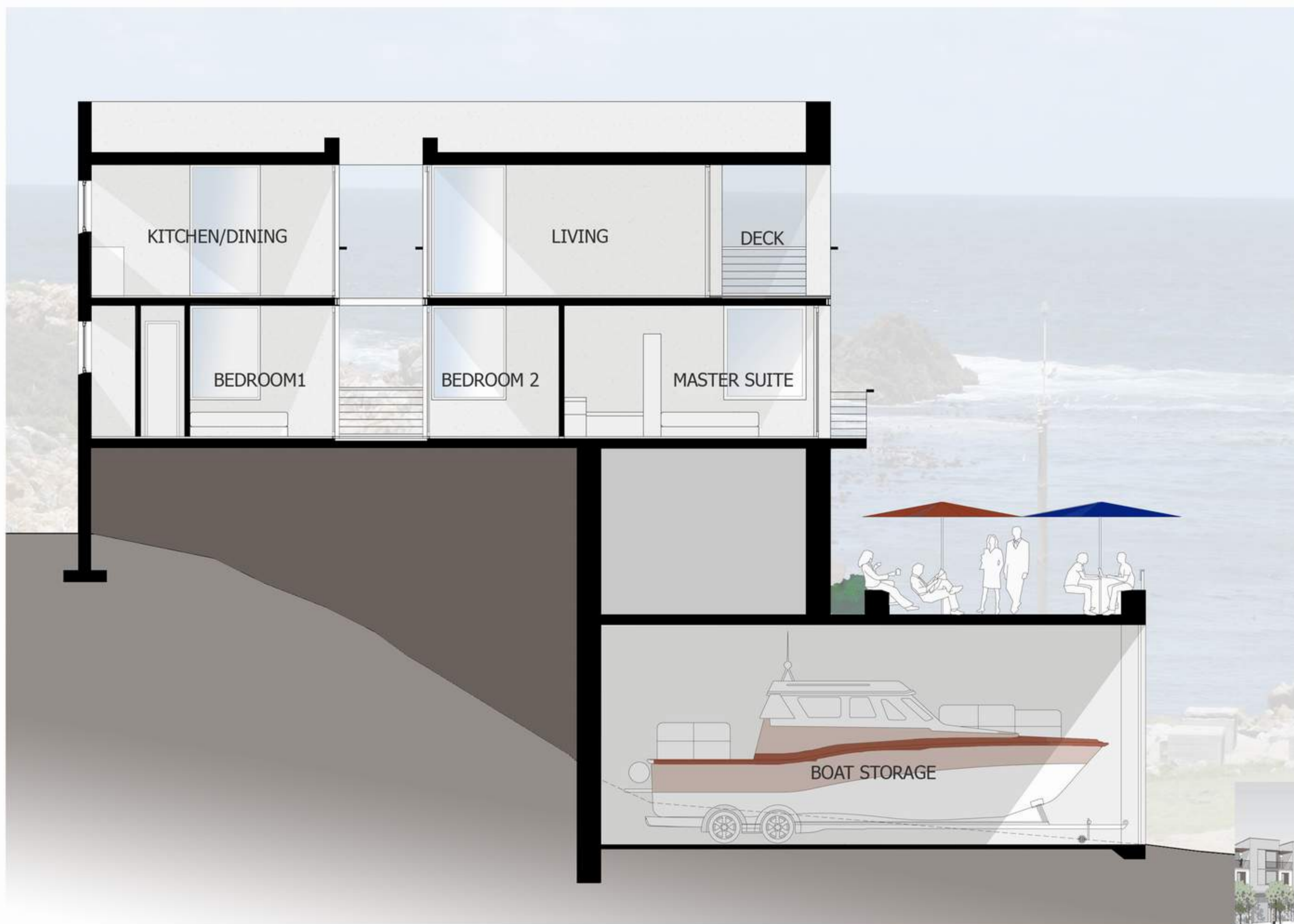
TYPICAL SECTION n.t.s.
